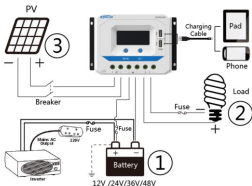
Obrázek 2 Schéma zapojení
