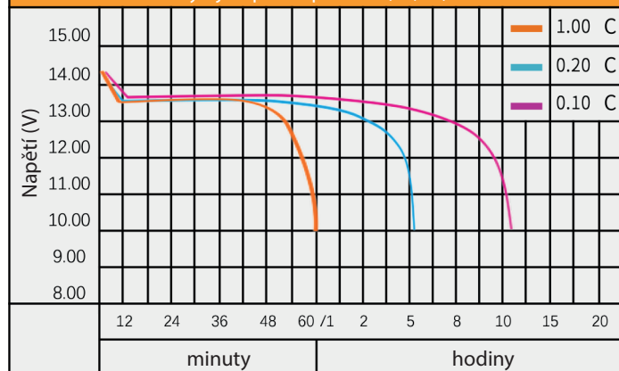
Vybíjecí proud při 25°C (12,8V)
