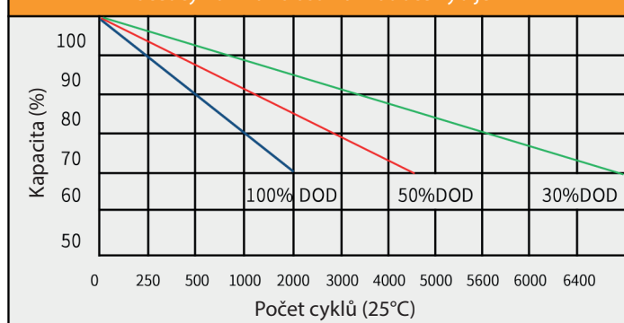
Počet cyklů v závislosti na hloubce vybíjení
