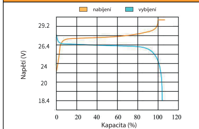
Nabíjecí a vybíjecí charakteristika (25,6V)
