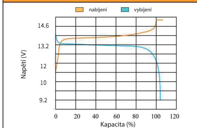
Nabíjecí a vybíjecí charakteristika (12,8V)
