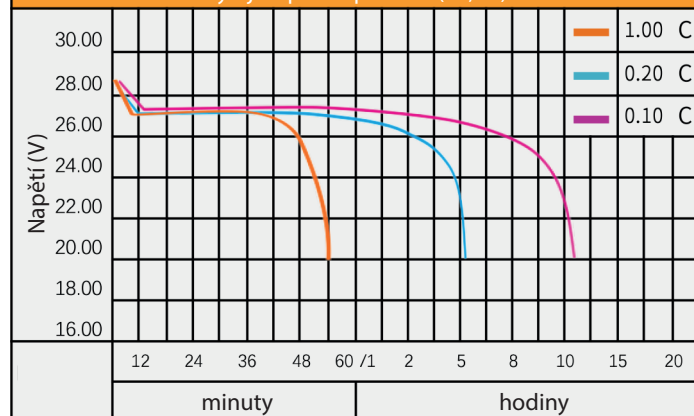
Vybíjecí proud při 25°C (25,6V)
