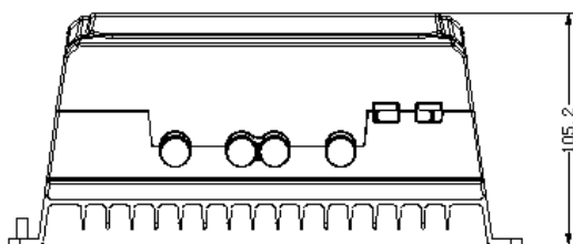
Tracer6210AN Rozměry (jednotka: mm)
